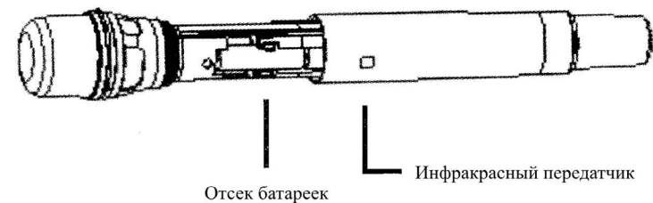
Задняя часть радиомикрофона
