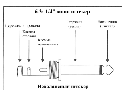
Небалансный штекер
